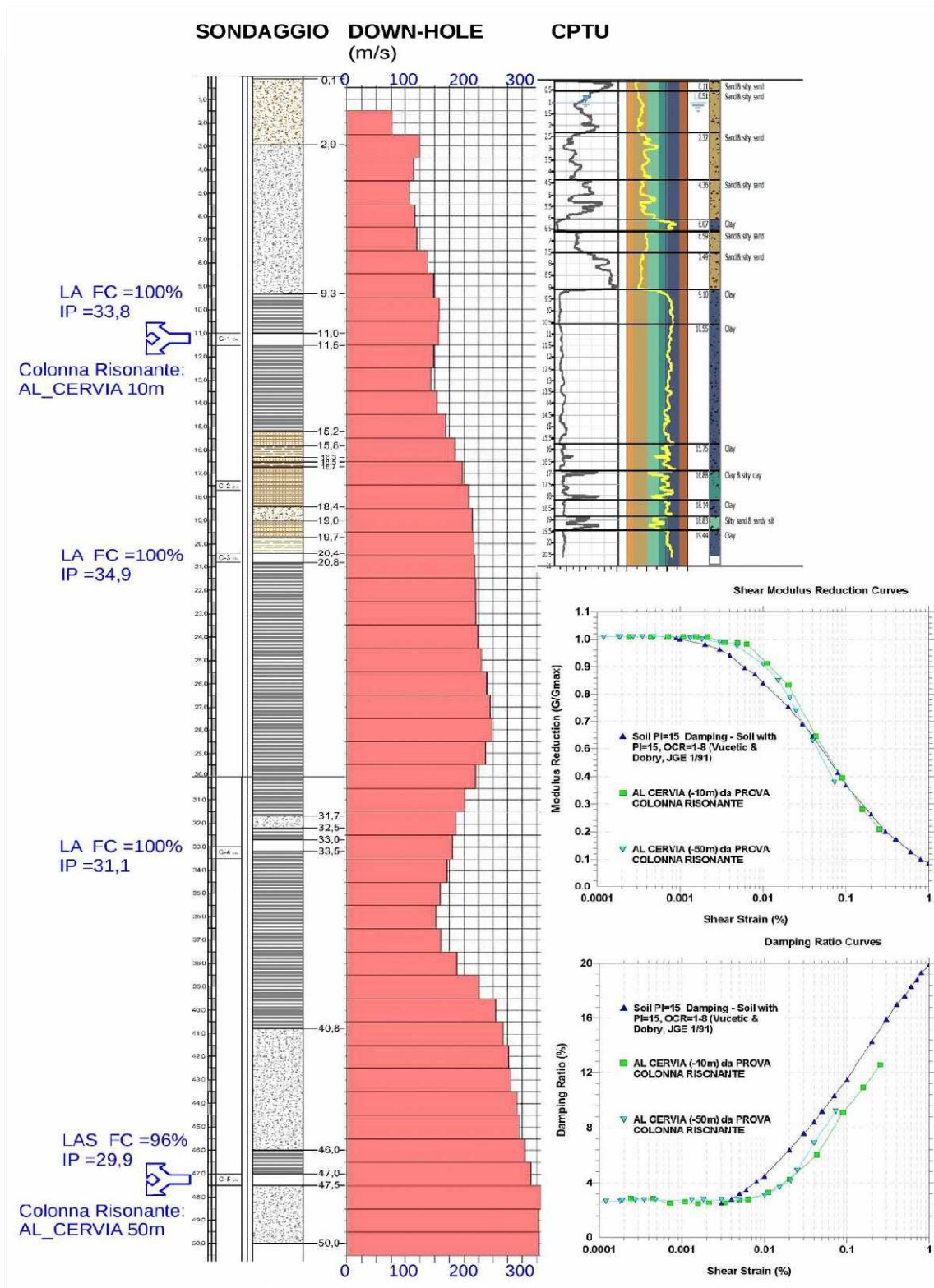
Figura 5.11 – Modellazione sismostratigrafica dei sedimenti investigati dal sondaggio/ “Down-Hole” eseguito per lo studio di microzonazione sismica a Pinarella di Cervia (nell’area verde tra via Donati e via Lazio). È riportato il confronto con la CPTU limitrofa. La figura riporta anche le curve di decadimento dei sedimenti fini di riferimento per le modellazioni numeriche della RSL del settore di costa cervese
