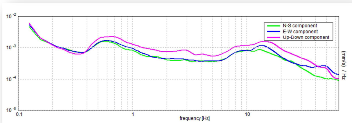
A: Curva H/V; B: Andamento componenti velocimetriche (E-W, N-S, Up-Down); C: Storia temporale H/V (le bande di colore nero corrispondono alle finestre di registrazione eliminate)
