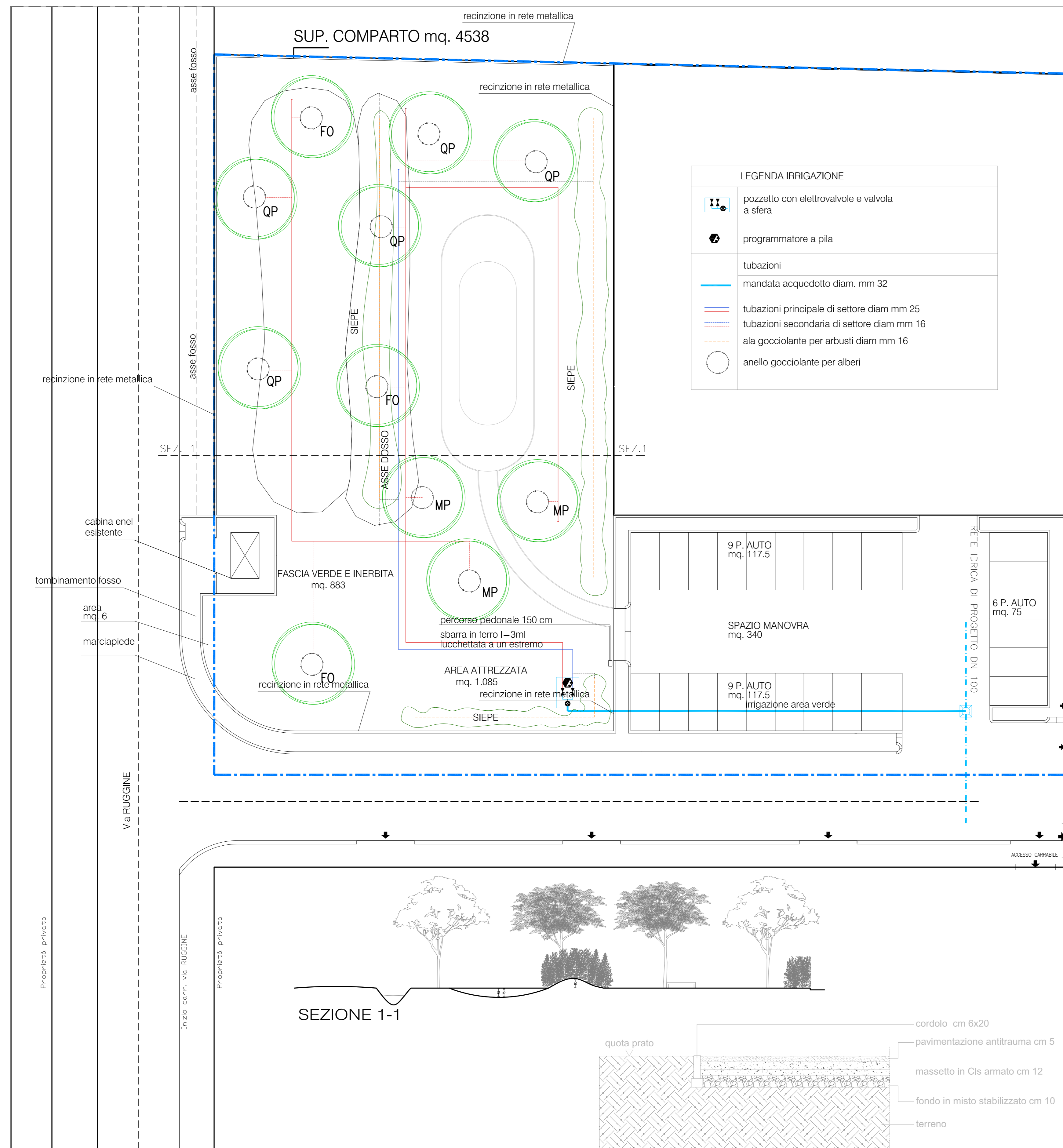
PLANIMETRIA DI PROGETTO SCALA 1:200
