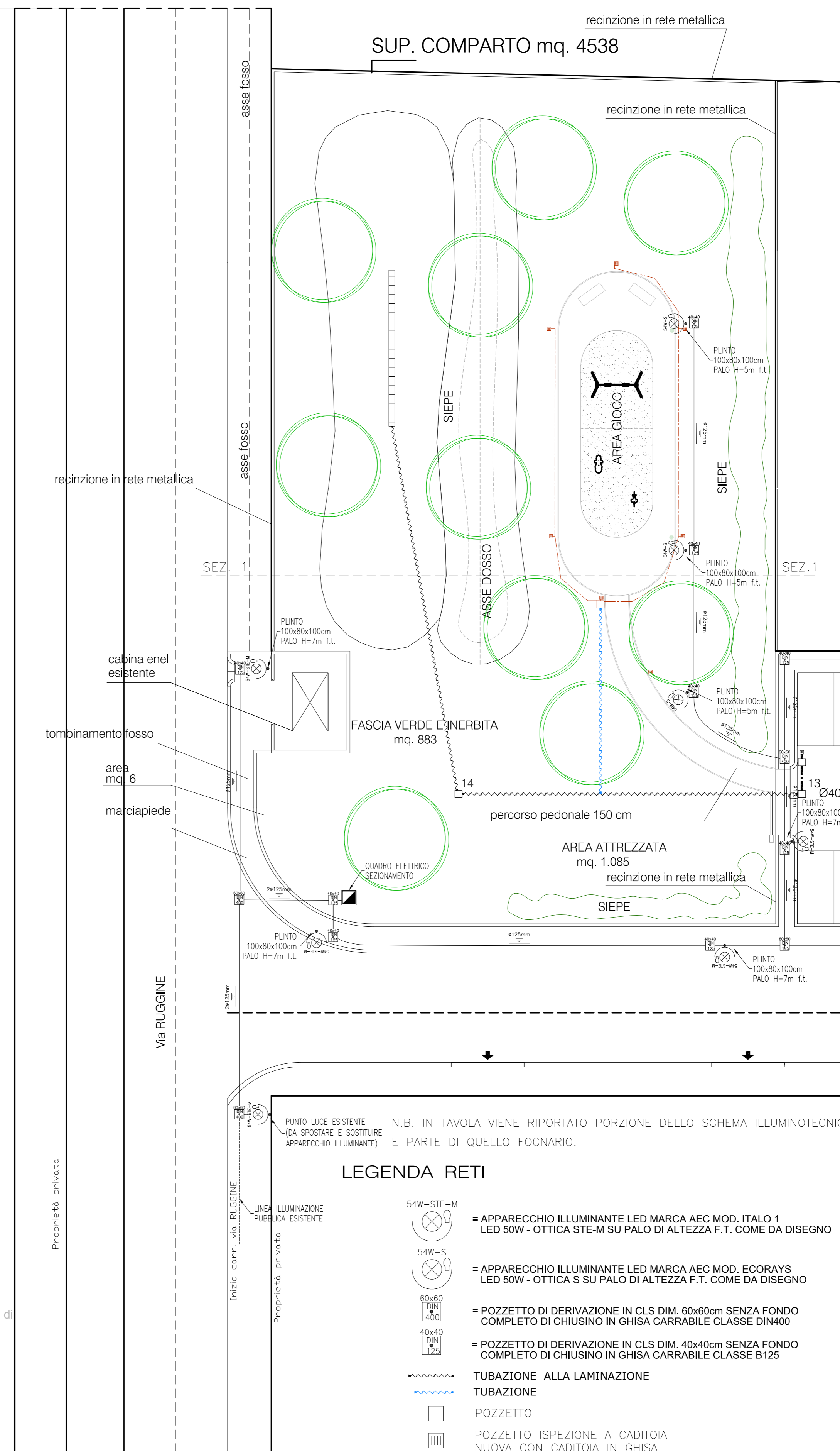
PLANIMETRIA DI PROGETTO SCALA 1:200
