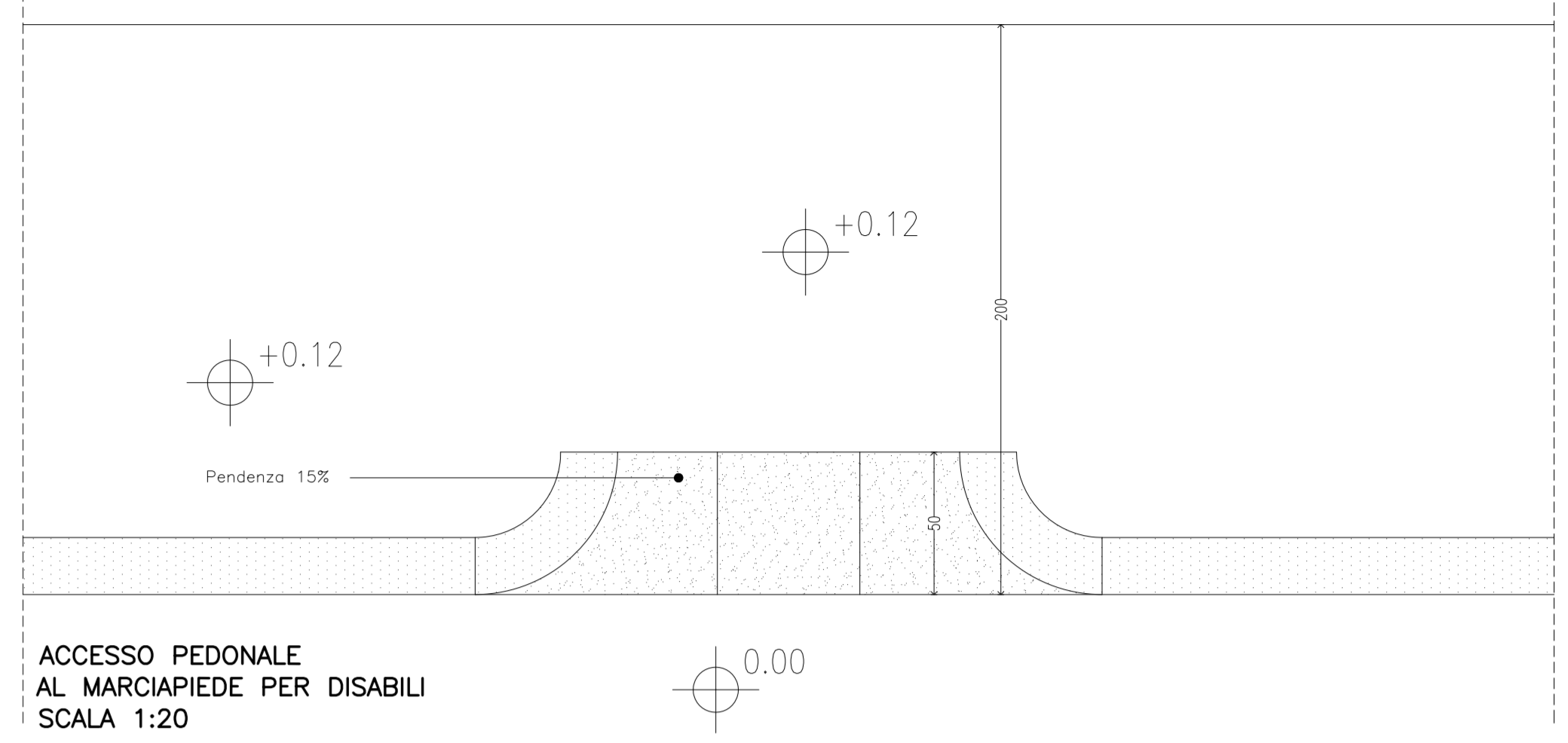
ACCESSO PEDONALE AL MARCIAPIEDE PER DISABILI SCALA 1:20
