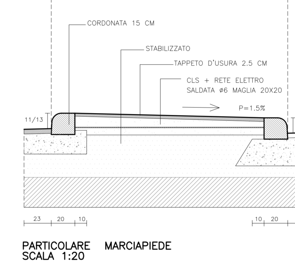
PARTICOLARE MARCIAPIEDE SCALA 1:20
