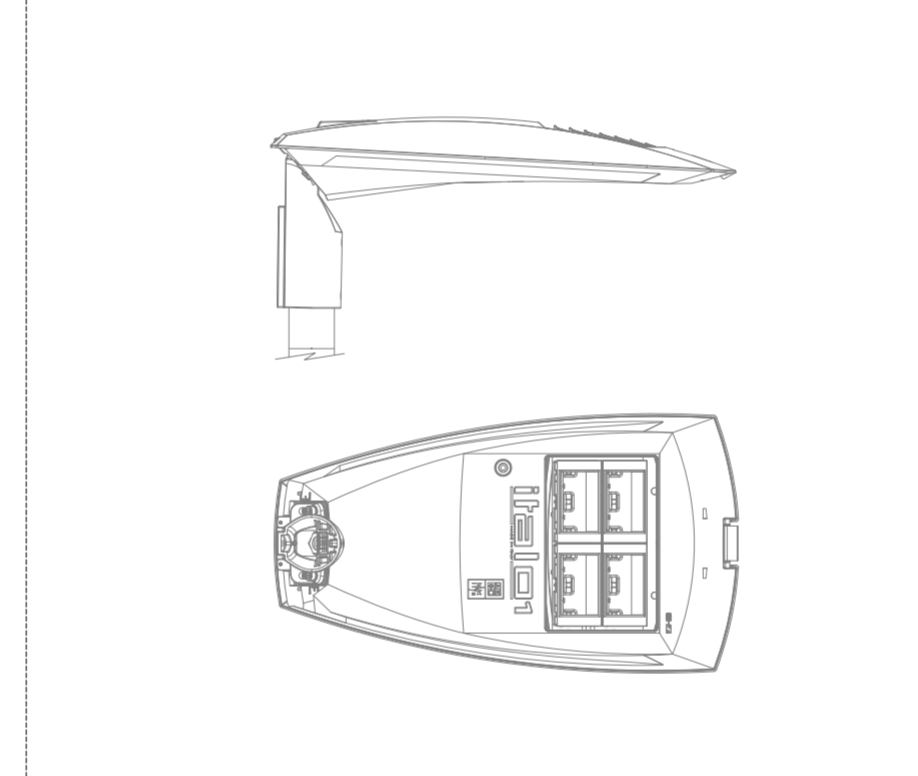
CORPO ILLUMINANTE LED MARCA AEC MOD. ITALO 1 LED - OTTICA STE-M
