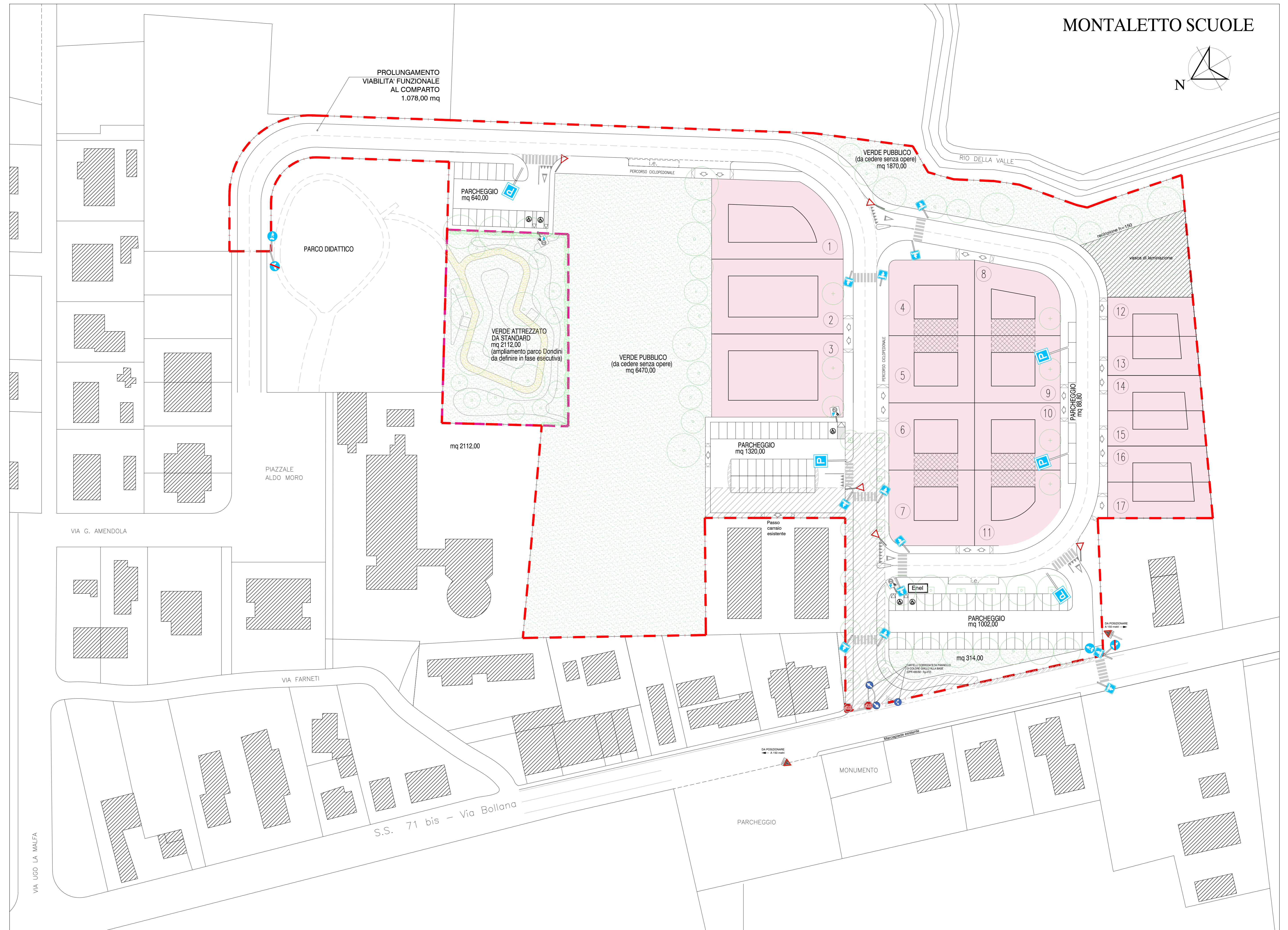
PLANIMETRIA 1:500
